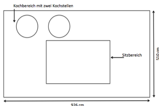
Abbildung 2: Skizze des Koch- und Essbereichs
